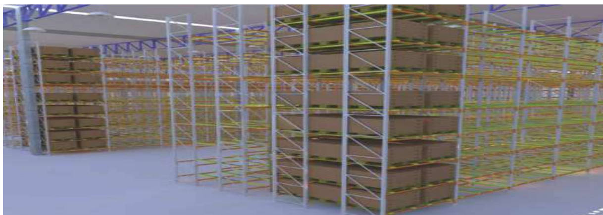
Figura 02 – Sistema de armazenagem por acumulação.
